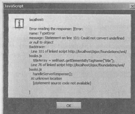
Рис. 2.10. Opera выводит очень подробные сообщения об ошибках
