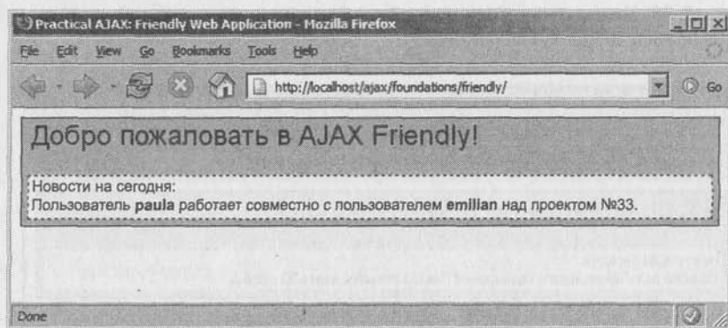
Рис. 3.21. Веб-приложение Friendly
