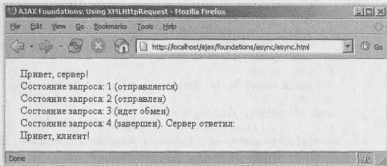
Рис. 2.6. Четыре кода состояния запроса
