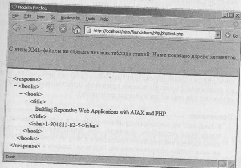
Рис. 3.1. Простой документ XML, сгенерированный PHP
