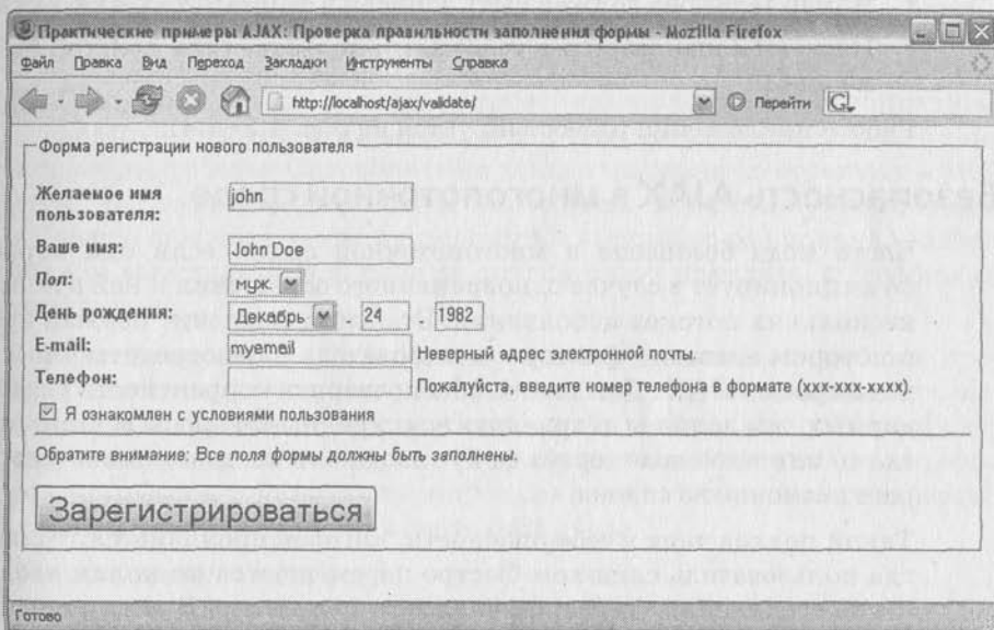
Рис. 4.3. Функция проверки правильности заполнения в действии
