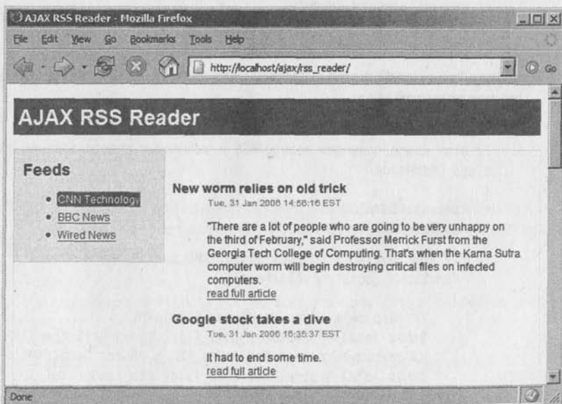
Рис. 9.2. Начальная страница нашего приложения чтения лент RSS
