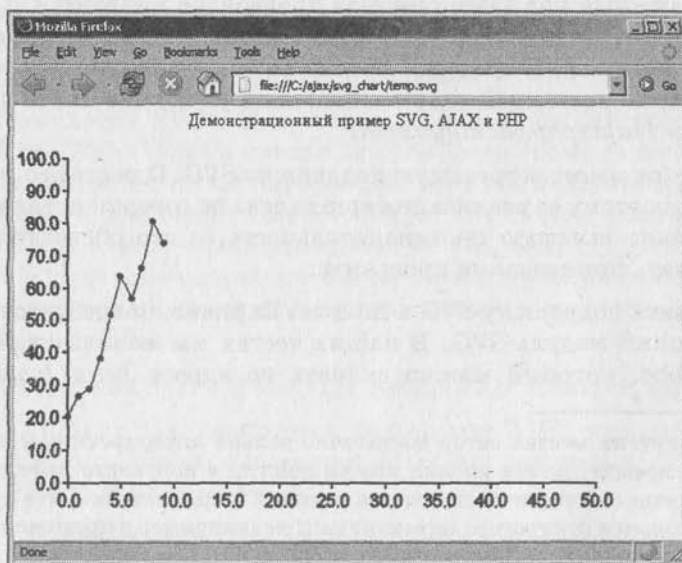
Рис. 7.1. Диаграмма SVG
